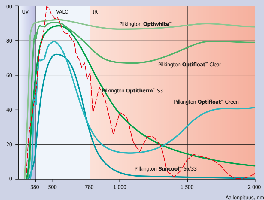
Aurinkoenergian läpäisy, %
